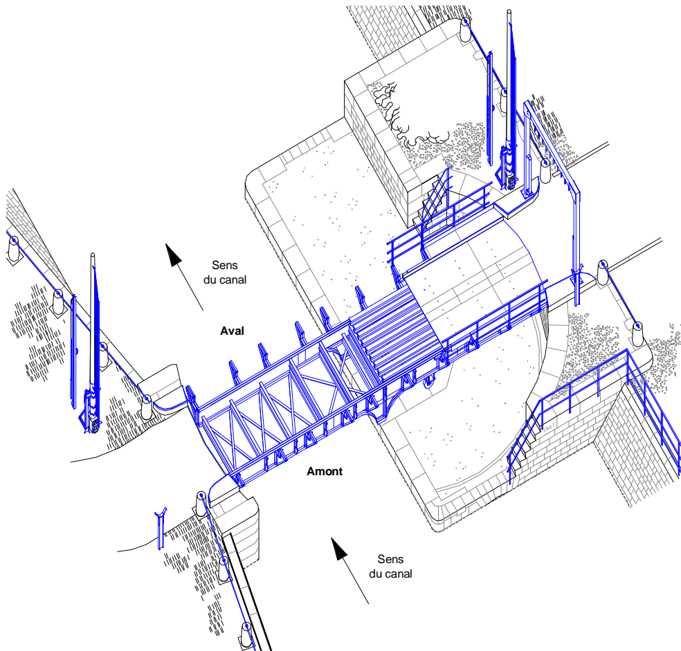
Axonométrie
