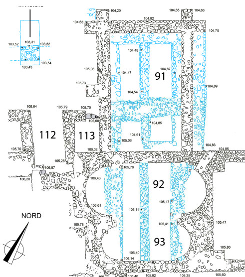
Plan des pièces 91, 92, 93, 112 et 113
