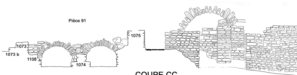
Coupe sur la pièce 91
