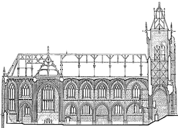
Coupe longitudinale
