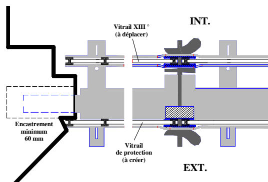
Détail de la mise en place d'une verrière de doublage
