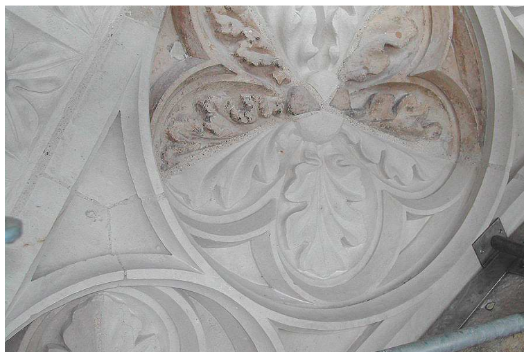
Restauration des polylobes sculptés, en cours de travaux Avant la mise en place du groupe sculpté du gâble
