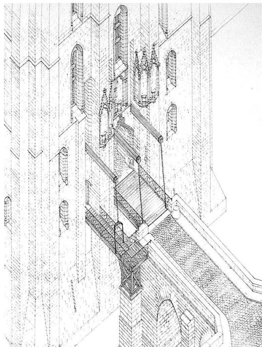
Axonométrie de l'état projeté réalisé
