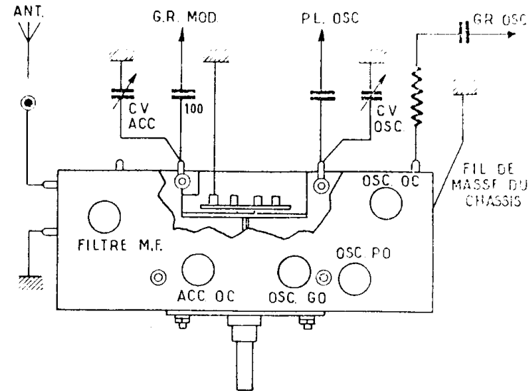
Bloc de bobinages du récepteur D925.
